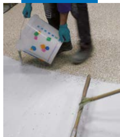
Gieten van Ultratop op het uitgehard oppervlak van het mengsel met natuurlijke aggregaten + Mapefloor I 910
